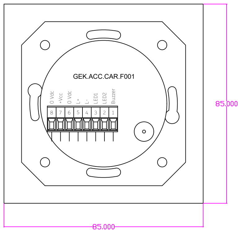
Zutritt RFID Lesegerät für Wand UP Montage, Schwarz T:13mm
