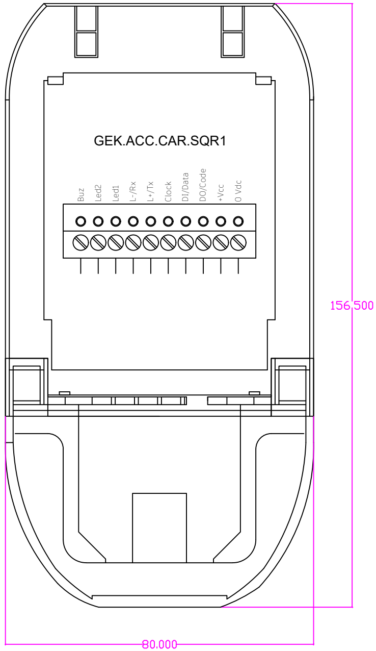
Zutritt RFID Lesegerät Aufputz mit QR-Code, Schwarz T:36mm
