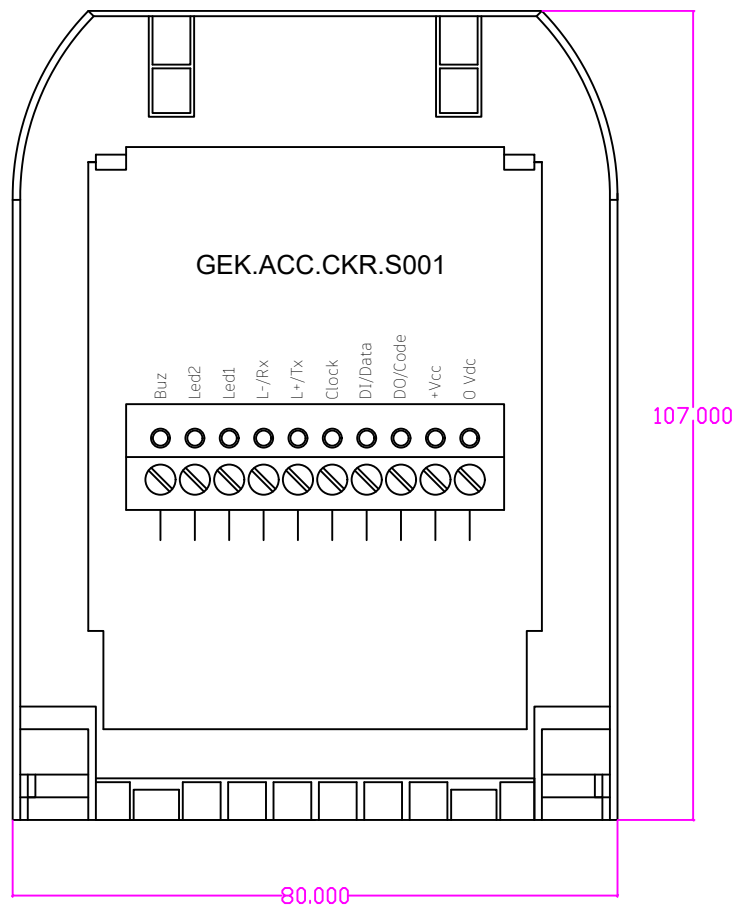
Zutritt RFID Lesegerät, Aufputz, mit Keypad, Schwarz T:25,6mm
