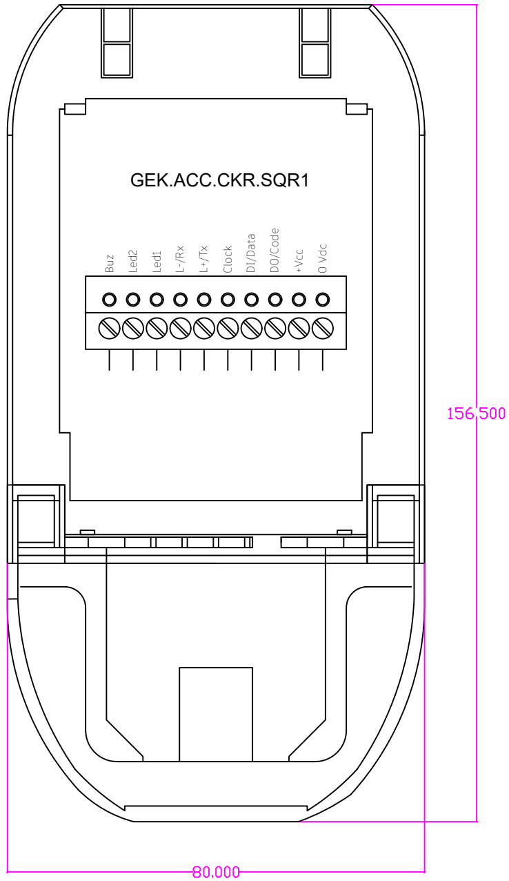
Zutritt RFID Lesegerät, Aufputz, mit Keypad und QR-Code T:36mm
