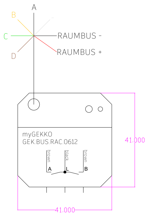
RAC RAUMBUS Unterputzaktor Beschattung T:22mm
