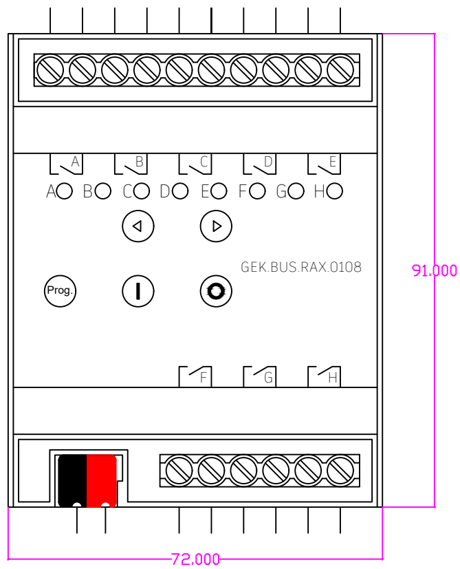
RAX RAUMBUS Aktor Hutschienenmontage 8DO T:62mm
