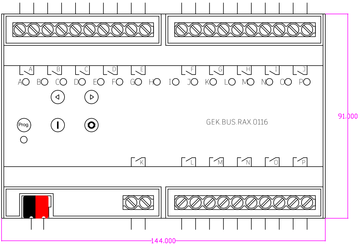
RAX RAUMBUS Aktor Hutschienenmontage 16DO T:62mm
