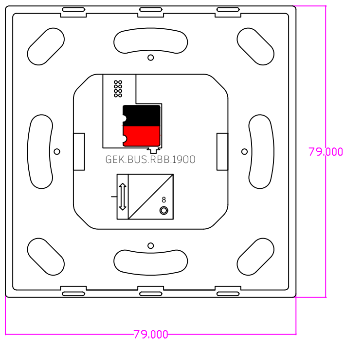
RAUMBUS 8-fach Taster, weiß T:35mm
