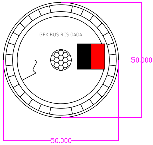
RCS04 RAUMBUS Mini Deckensensor T:19mm
