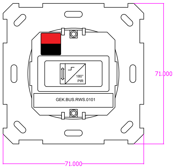
RWS01 RAUMBUS Wand Bewegungssensor 180° T:15 mm
