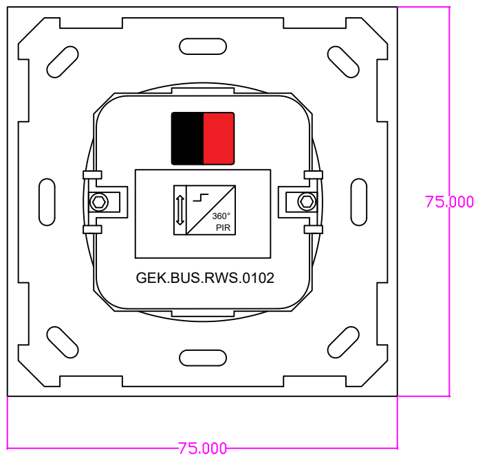
RWS01 RAUMBUS Decken Präsenz- und Bewegungssensor 360° T:35mm
