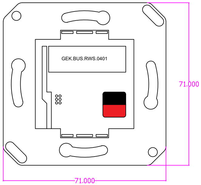
RWS04 RAUMBUS Raumsensor Temperatur, Weiß, 55x55 (Fenster) T:15mm
