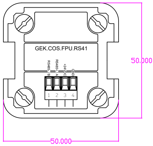
FPU Fingerprint Unterputz für 55x55 Einbau T:30,5mm
