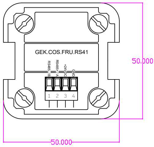
FRU Fingerprint mit RFID Unterputz für 55x55 Einbau T:30,5mm
