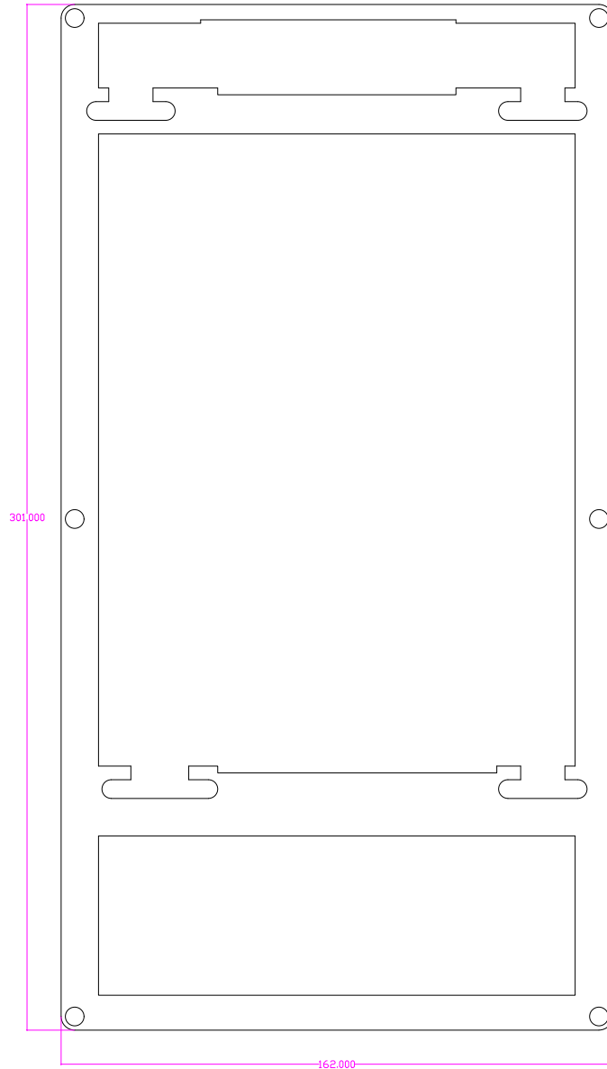
Einschubhalterahmen für myGEKKO SLIDE2
