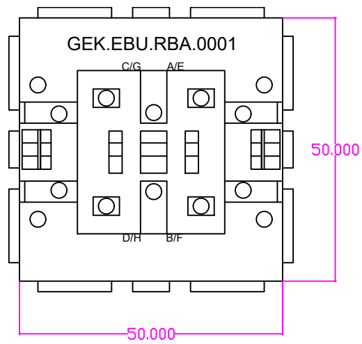
RBA 00 myGEKKO Tasteraufsatz 4-fach, ohne Wippen
