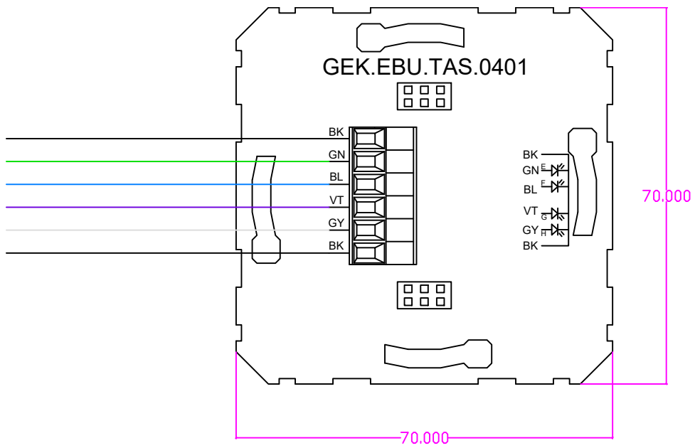
TAS 04 UP Zusatztaster 4fach 55x55 mm, 24 V ohne Wippen
