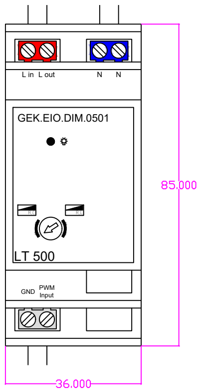
PWM Lichtdimmer 500VA T: 77mm
