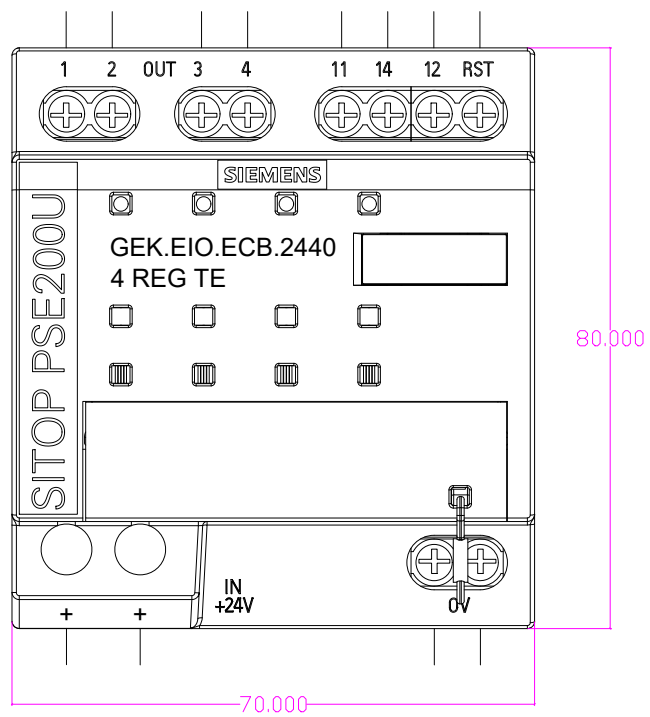
SITOP PSE200U 3 A Selektivitätsmodul 4-kanalig T:70mm
