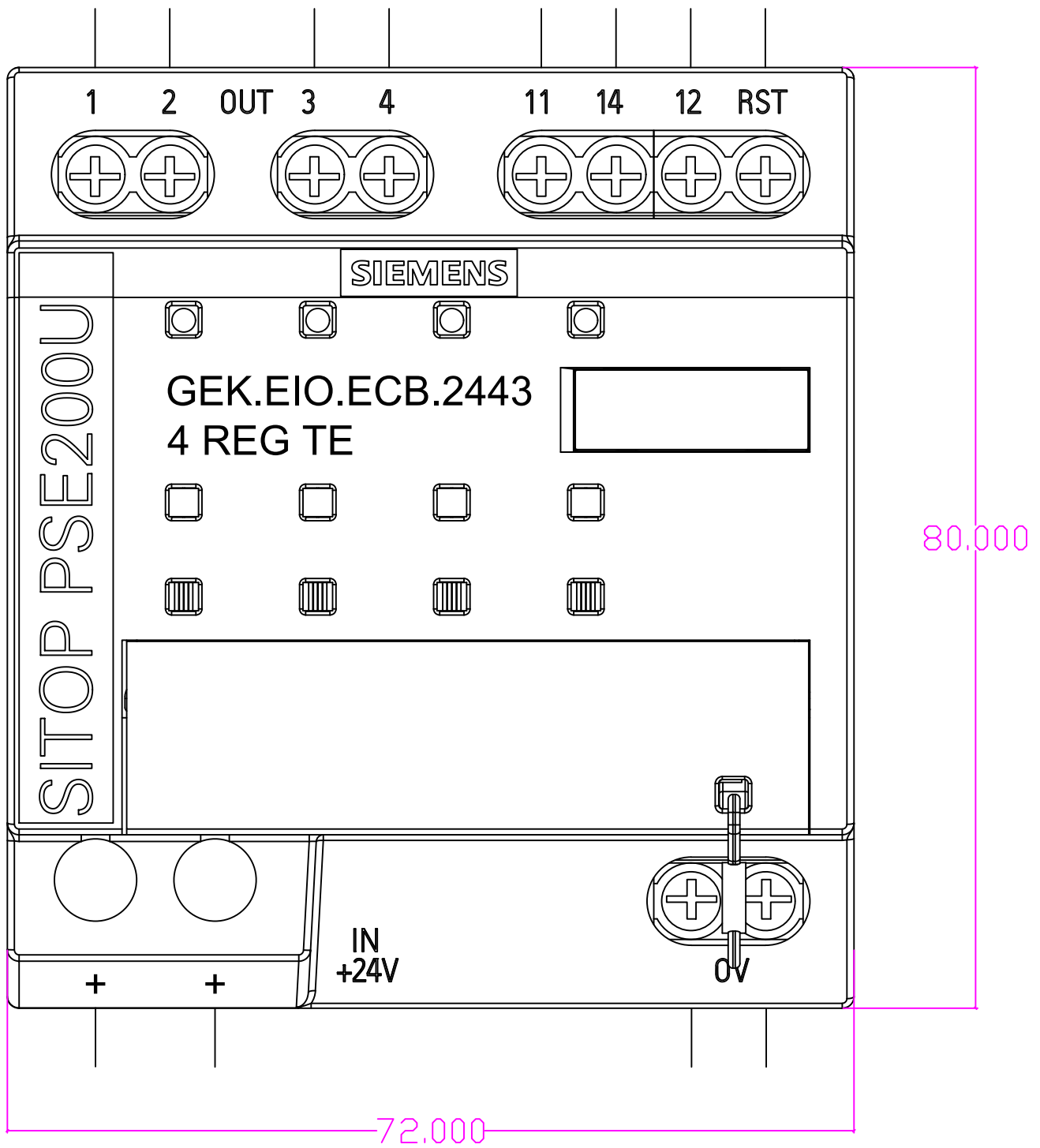
SITOP PSE200U 0.5 bis 3A Selektivitätsmodul 4-kanalig T:70mm
