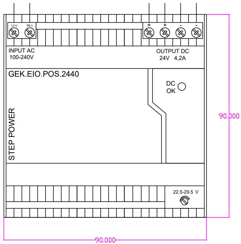
Spannungsversorgung REG 4,2 A bei 24 V DC 5 REG TE T.60mm
