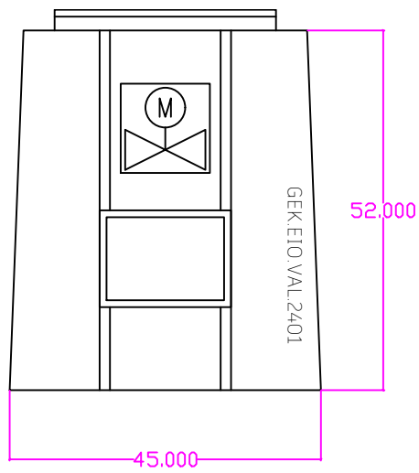
Thermoventilantrieb 24VDC inkl. Adapter(Gewinde: M30) & Kabel
