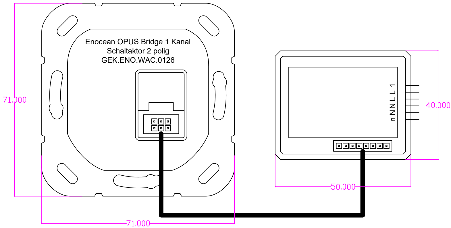
Enocan OPUS Bridge 1 Kanal Aktor 2 polig T=35mm
