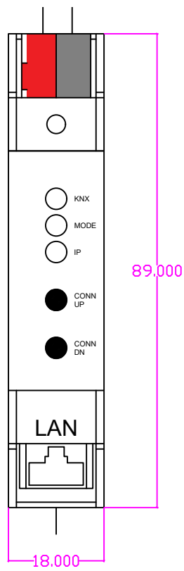
RAB LAN zu RAUMBUS Schnittstelle T:60mm
