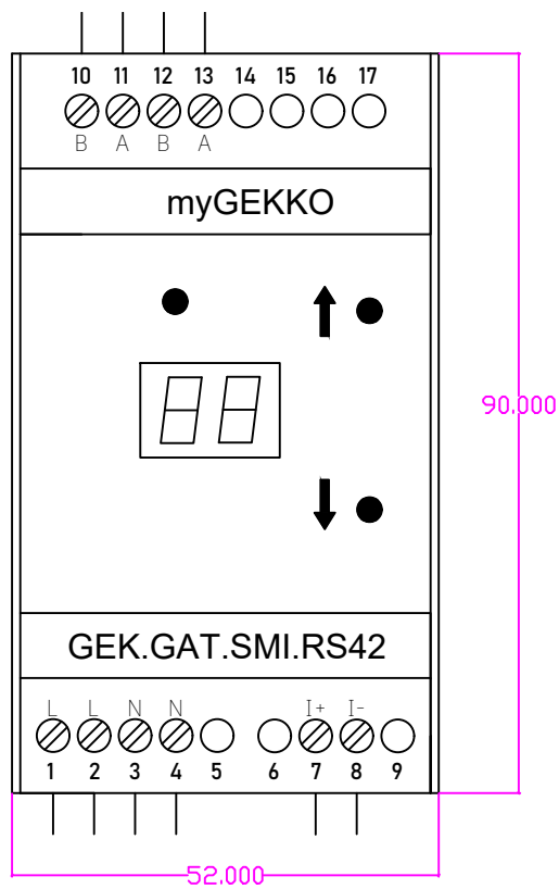
SMI RS485-SMI Schnittstelle REG-Einbau T:60mm REG 3TE
