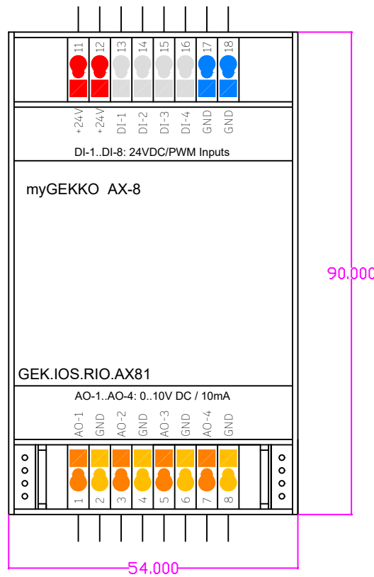
myGEKKO RIOAX8 Extendermodul für REG Einbau T:62mm REG 4TE
