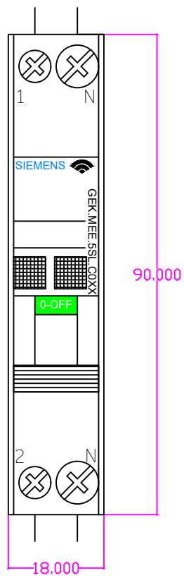
Leitungsschutzschalter 5SL6 COM mit Messfunktion als Energiezähler B - Charakteristik T:70mm
