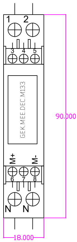
Einphasen Energiezähler 32A M-Bus T:63mm
