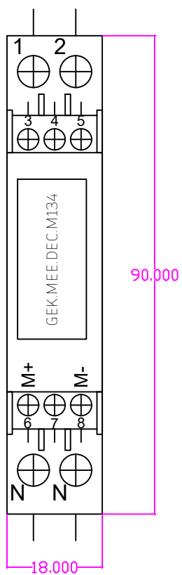
Einphasen Energiezähler 32A M-Bus, MID T:63mm
