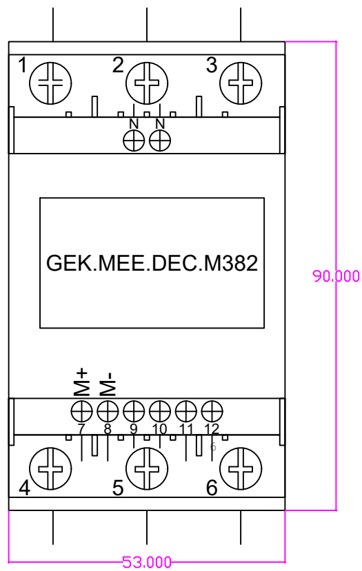
Dreiphasen Energiezähler 65A M-Bus, MID T:63mm
