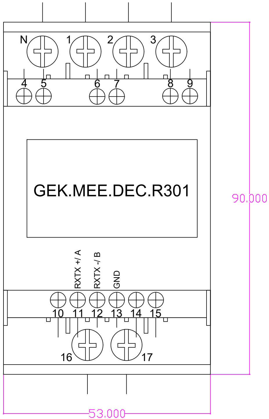
Dreiphasen Energiezähler 5A RS485 T:63mm
