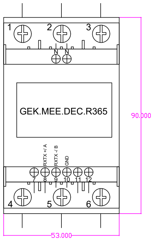
Dreiphasen Energiezähler 65A ModBus, RS485 T:63mm
