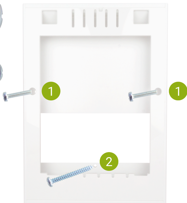
Abbildung 3: Montage/Schraubpunkte
